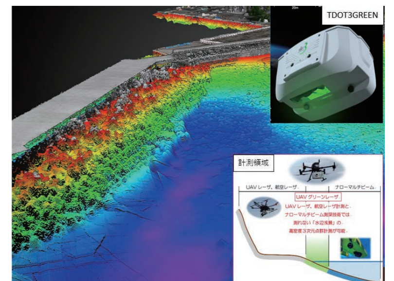
グリーンレーザ計測による水辺浅瀬の3次元点群データ
